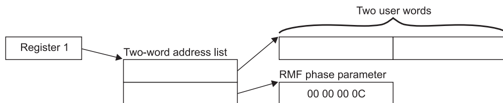
Figure 20. ERBMFTUR Input Parameter Structure
